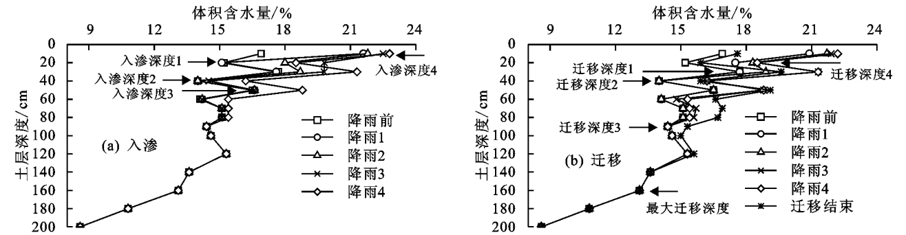
图 5 典型间歇降雨下土壤剖面水分变化
