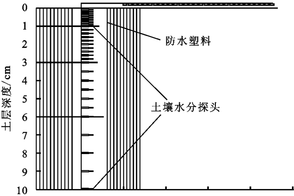
图 3 土壤水分探头布置
