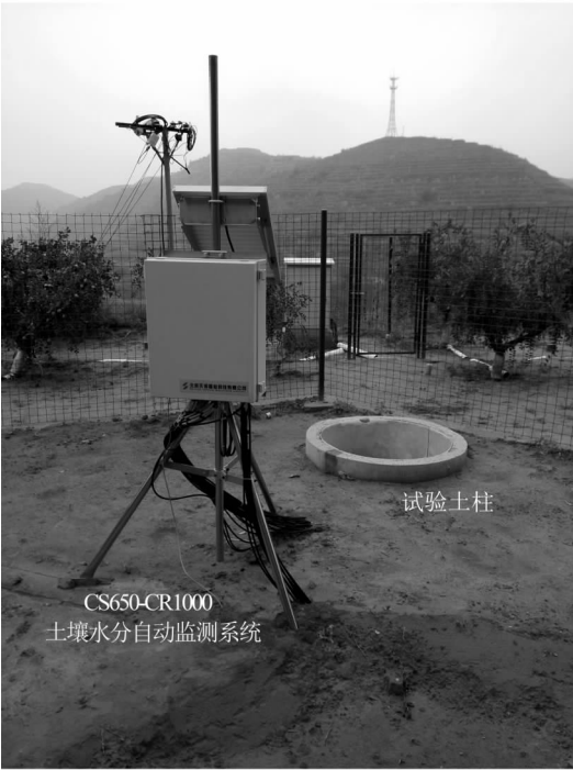
图 1 野外土柱布设状况
