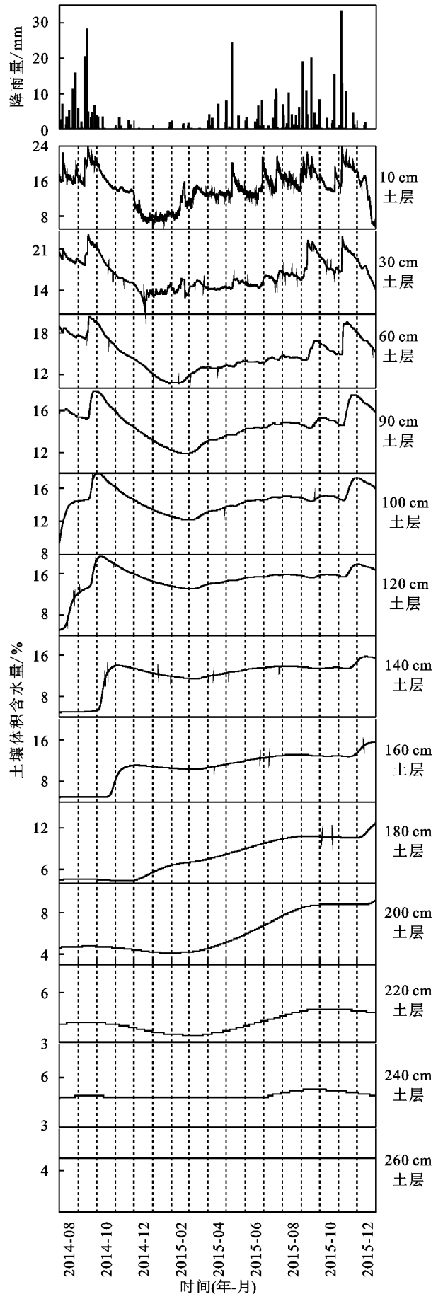
图 6 研究区降雨分配及土壤剖面水分变化状况
