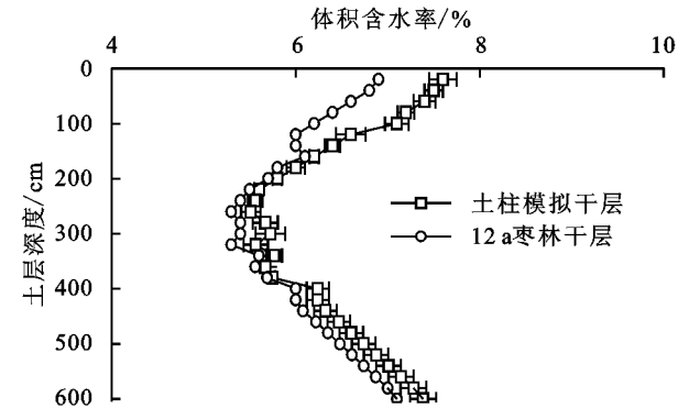
图 2 土柱模拟干层和 12 a 枣林实测干层土壤水分
