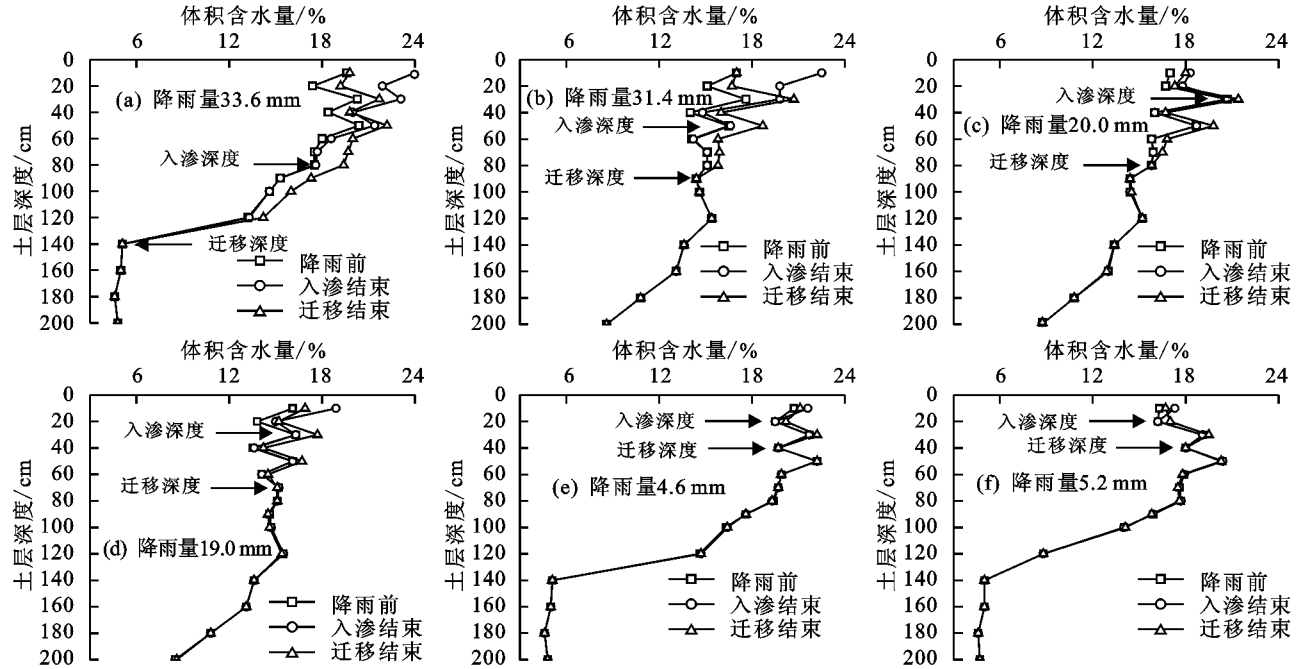
图 4 典型独立降雨下土壤剖面水分变化
